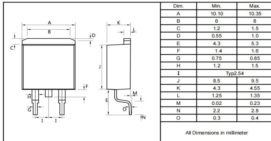
TO-263
